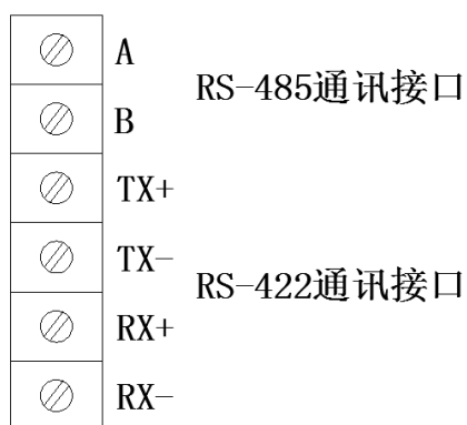
图 3-3 端子通讯口
