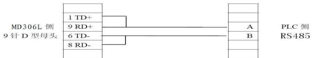
图 3-13 文本通讯线
